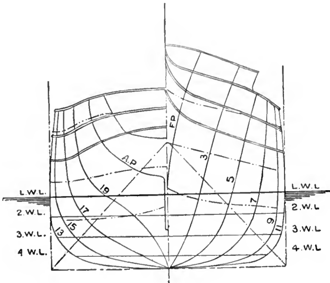
FIG. 87.—BODY PLAN.
